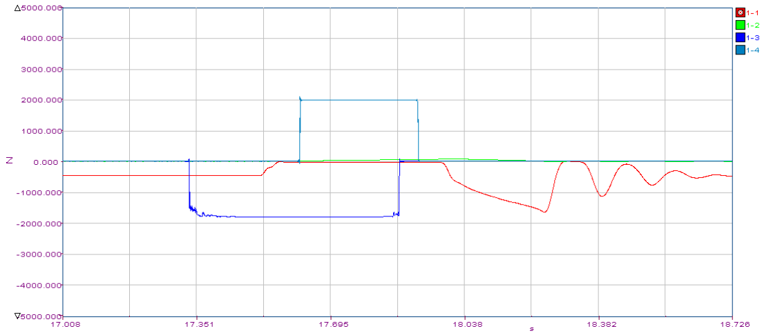
(5) 最终检验的试验速度工况测试数据曲线图
